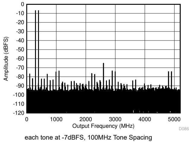
图 6-11. DES Mode: Two Tone FFT at 347MHz
