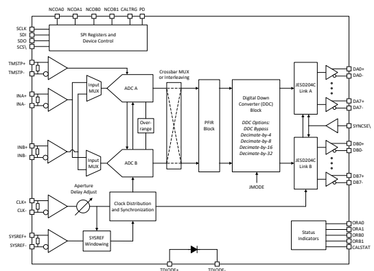
ADC12DJ5200RF 方框图
