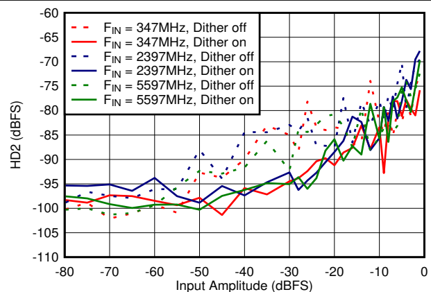
图 6-62. DES Mode: HD2 vs Input Amplitude and Dither
