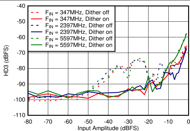
图 6-64. DES Mode: HD3 vs Input Amplitude and Dither
