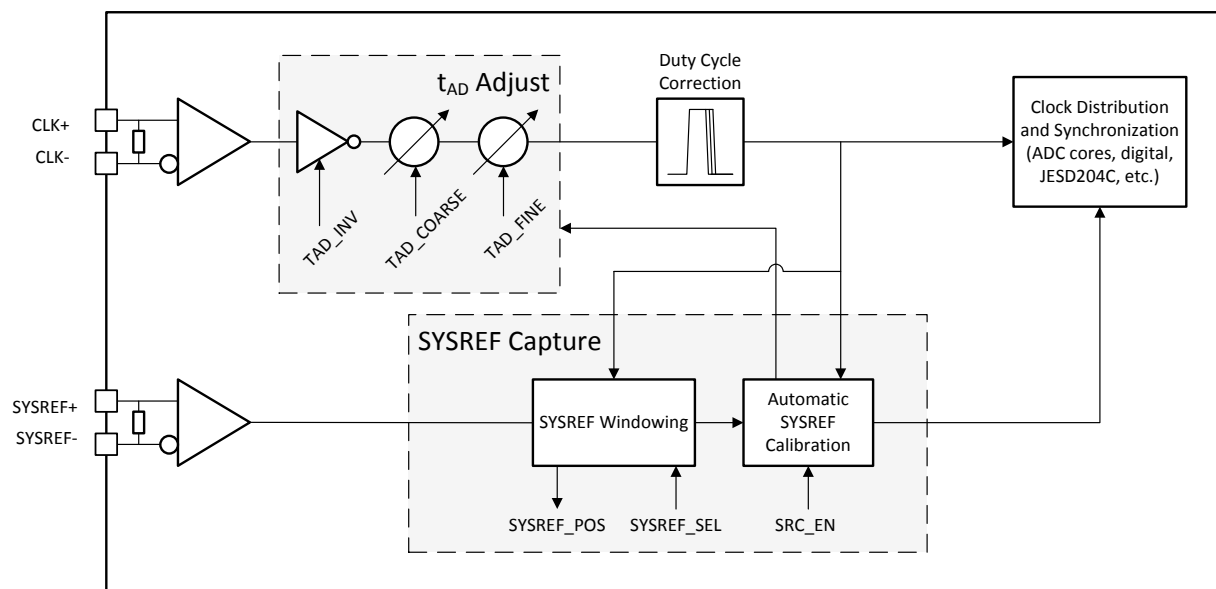
图 7-2. Clocking Subsystem
