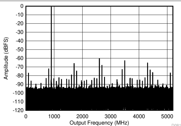
图 6-6. DES Mode: Single Tone FFT at 897MHz
