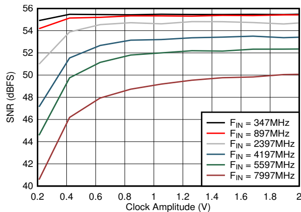
图 6-81. DES Mode: SNR vs Clock Amplitude
