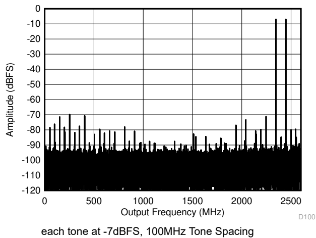
图 6-25. DES Mode: Two Tone FFT at 2397MHz
