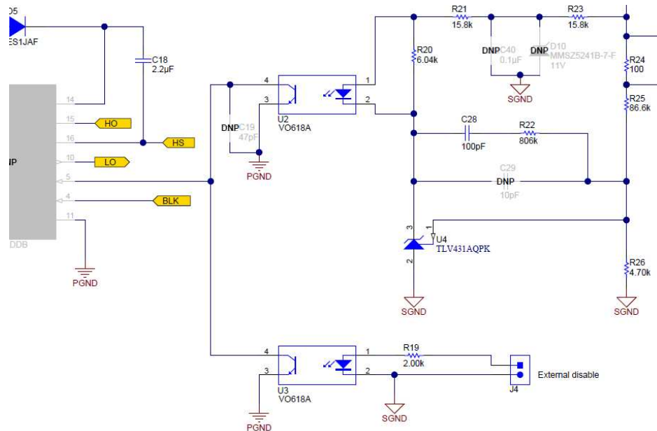
图 32. 外部禁用示例电路
