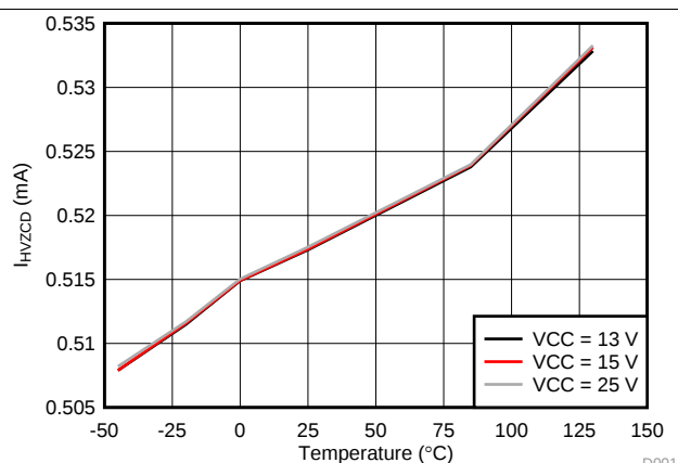
图 19. I_{HVZCD} 与温度间的关系
