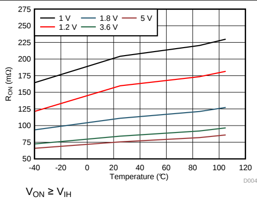
图 3. ON-Resistance ( R_{ON} )
