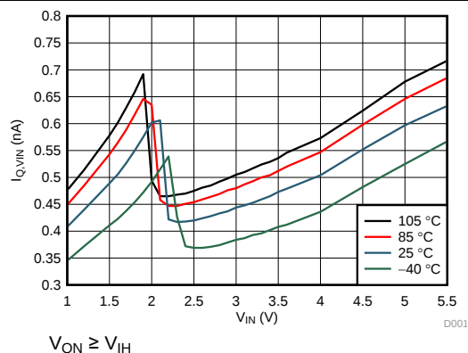
图 2. Quiescent Current ( I_Q )
