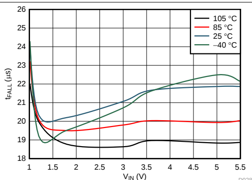
图 27. Turn Off Time
