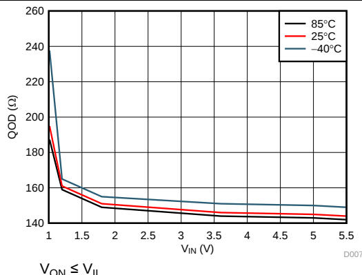
图 4. Quick Output Discharge (QOD)
