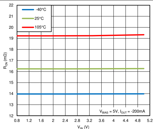
图 8. R_{ON} vs. V_{IN} ( V_{BIAS} = 5 V, Single Channel)
