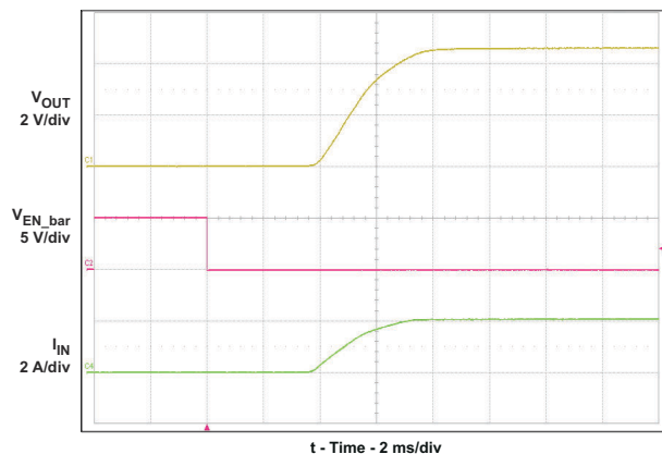
图 10-3. Turnon Delay and Rise Time
