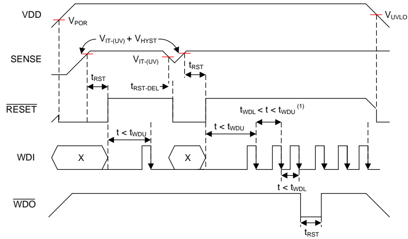
图 1. Timing Diagram
