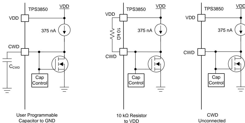
图 29. CWD Charging Circuit
