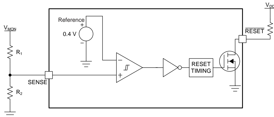
图 30. Adjustable Voltage Divider
