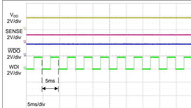
图 36. 200-Hz WDI Pulse
