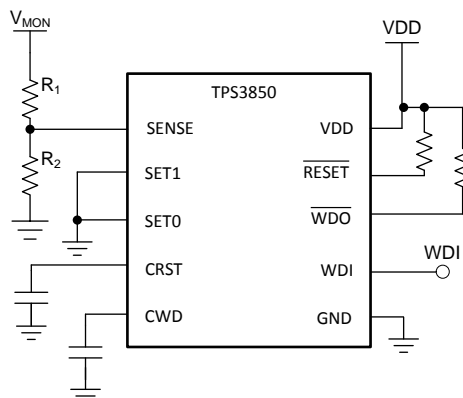
图 24. Adjustable Voltage Monitor
