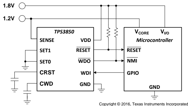
全集成微控制器监控电路
