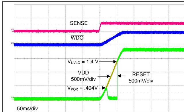
图 34. Startup Waveform
