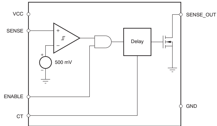
图 19. TPS3897A Block Diagram
