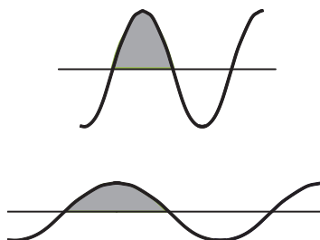
图 31. BEMF Integration
