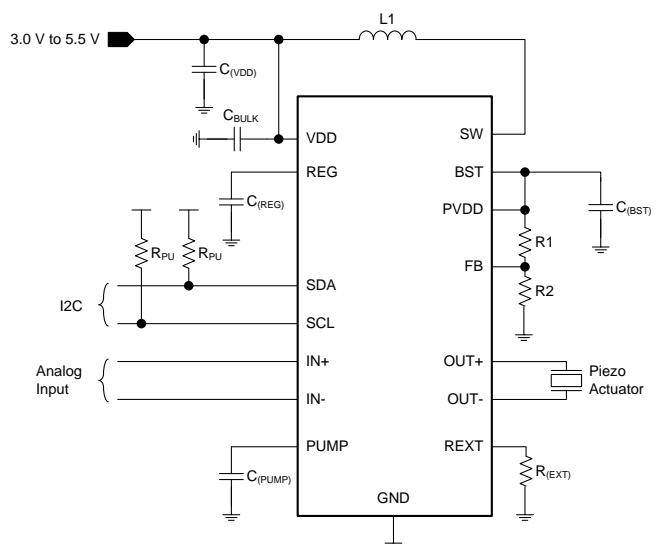
简化原理图
