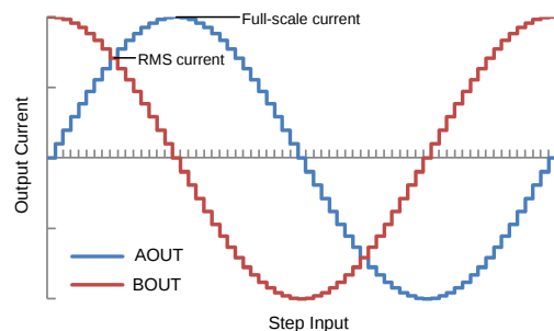
微步进电流波形
