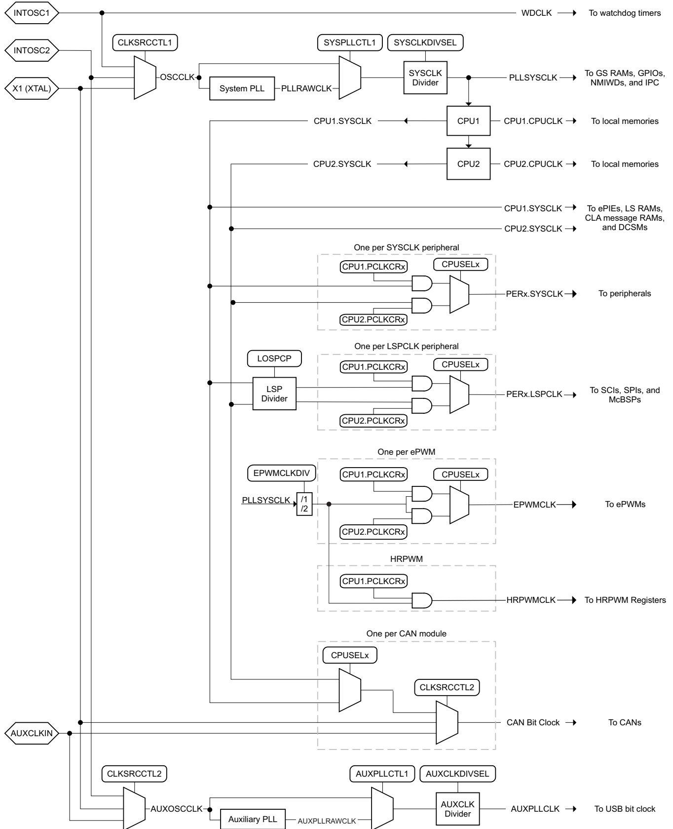
图 4-8. Clocking System
