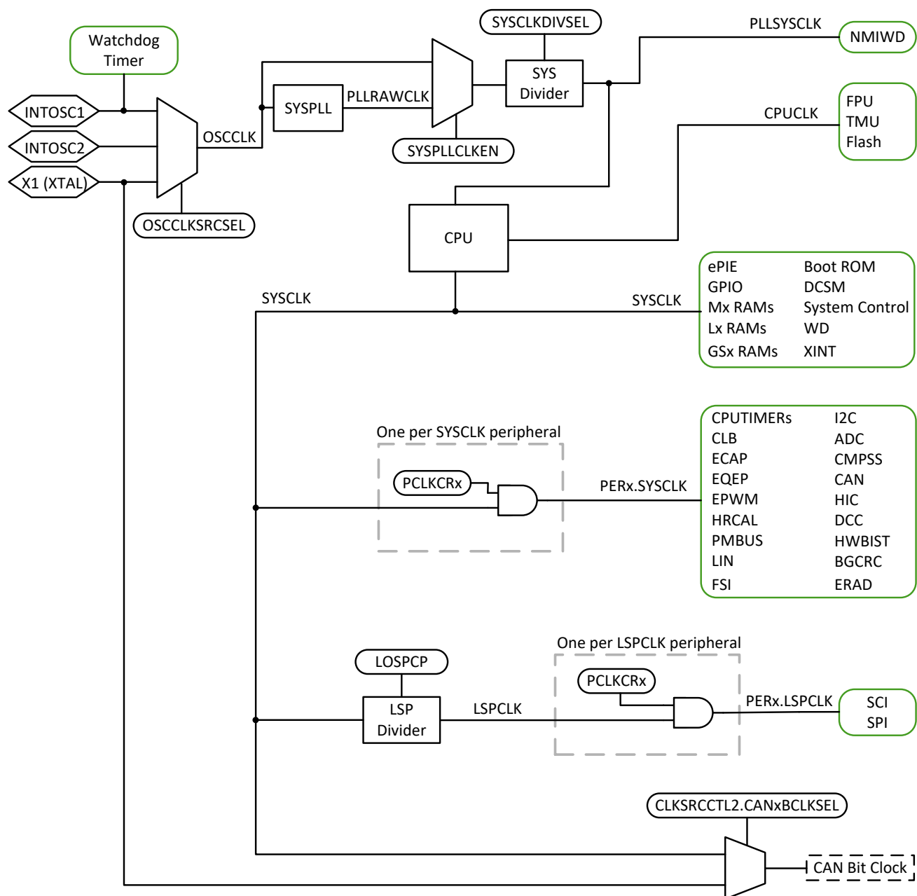
图 7-10. Clocking System
