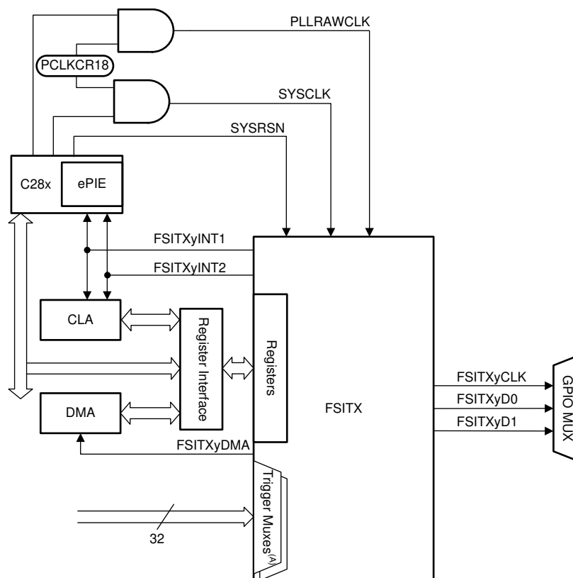
图 5-84. FSITX CPU Interface
