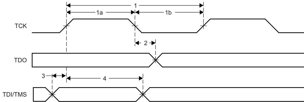
图 5-19. JTAG Timing
