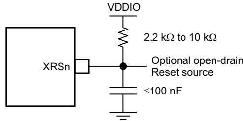
图 5-7. Reset Circuit
