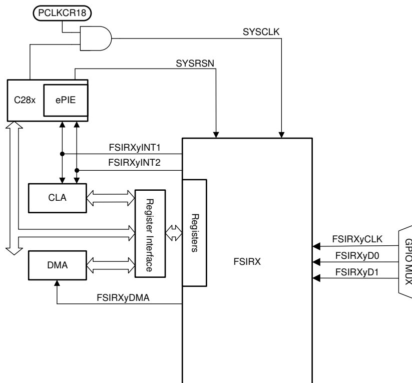
图 5-87. FSIRX CPU Interface
