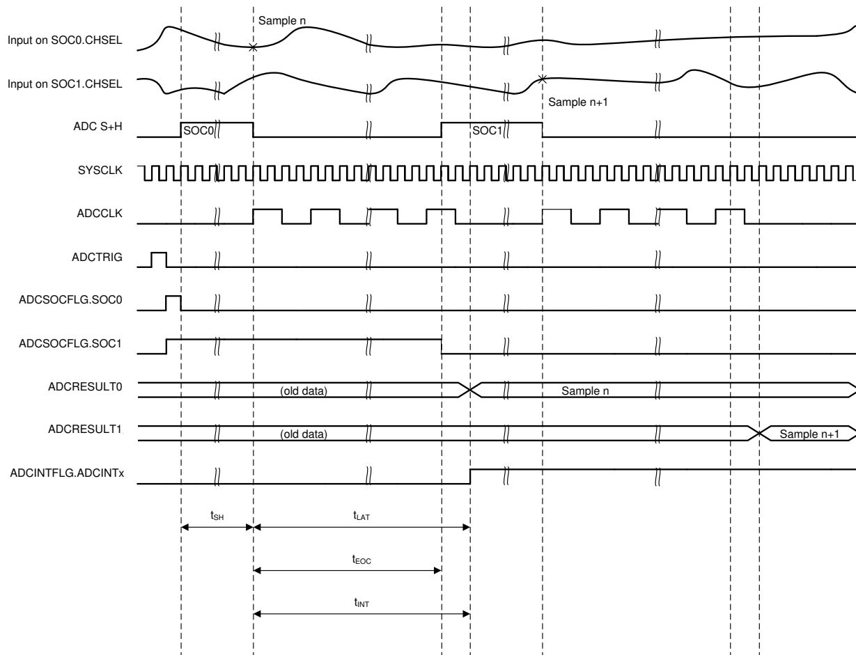
图 5-35. ADC Timings
