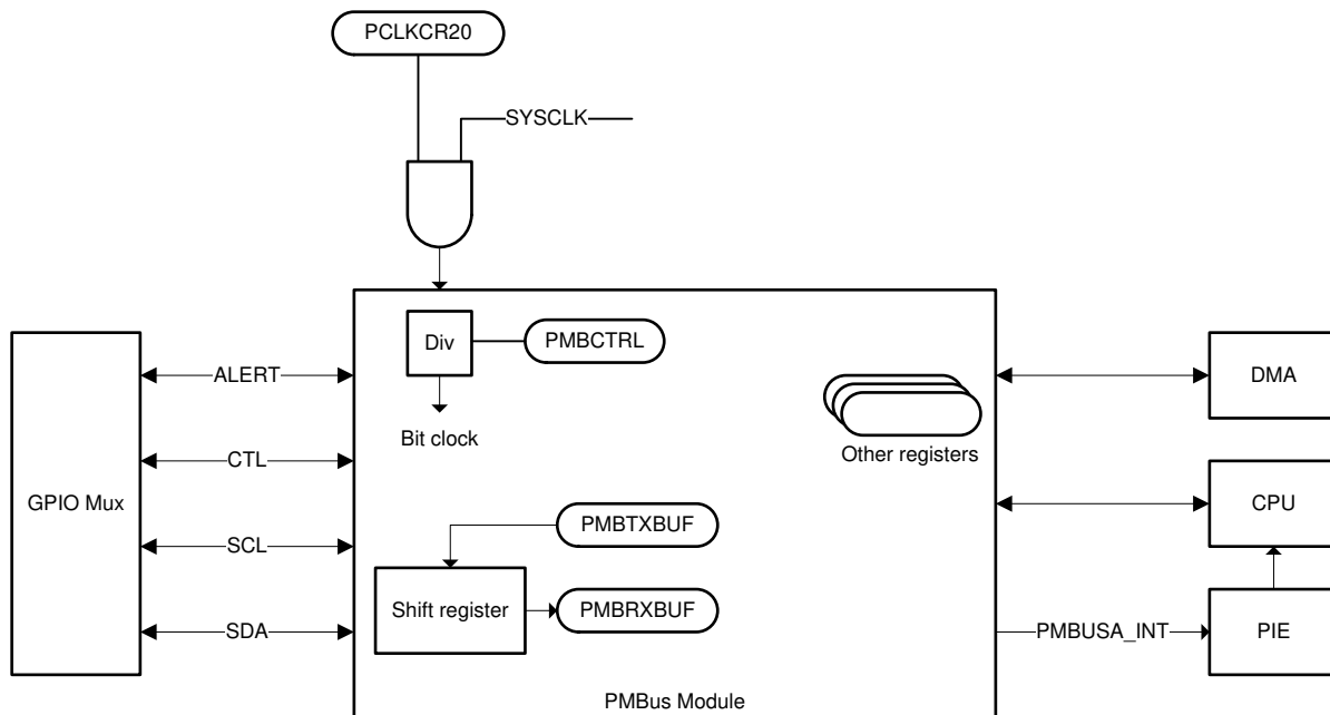
图 5-72. PMBus Block Diagram
