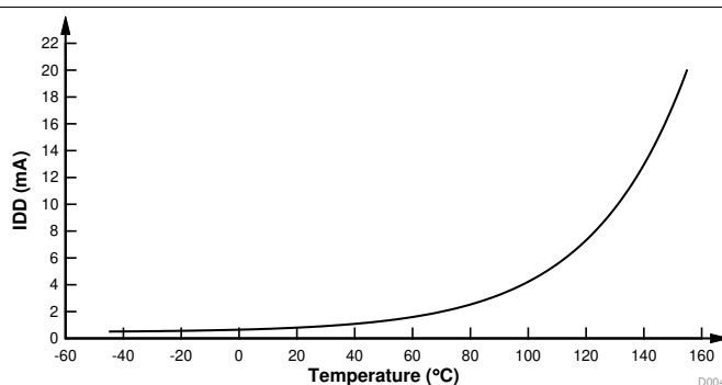
图 5-5. Halt Current Versus Temperature (°C)
