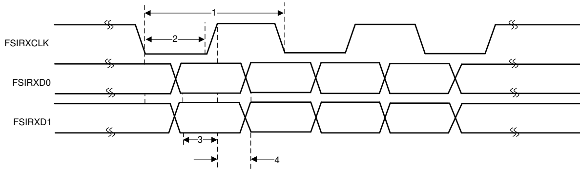
图 5-89. FSIRX Timings
