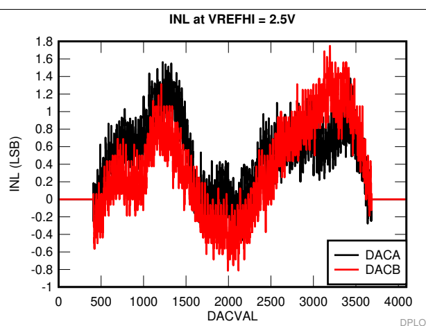
图 5-43. INL
