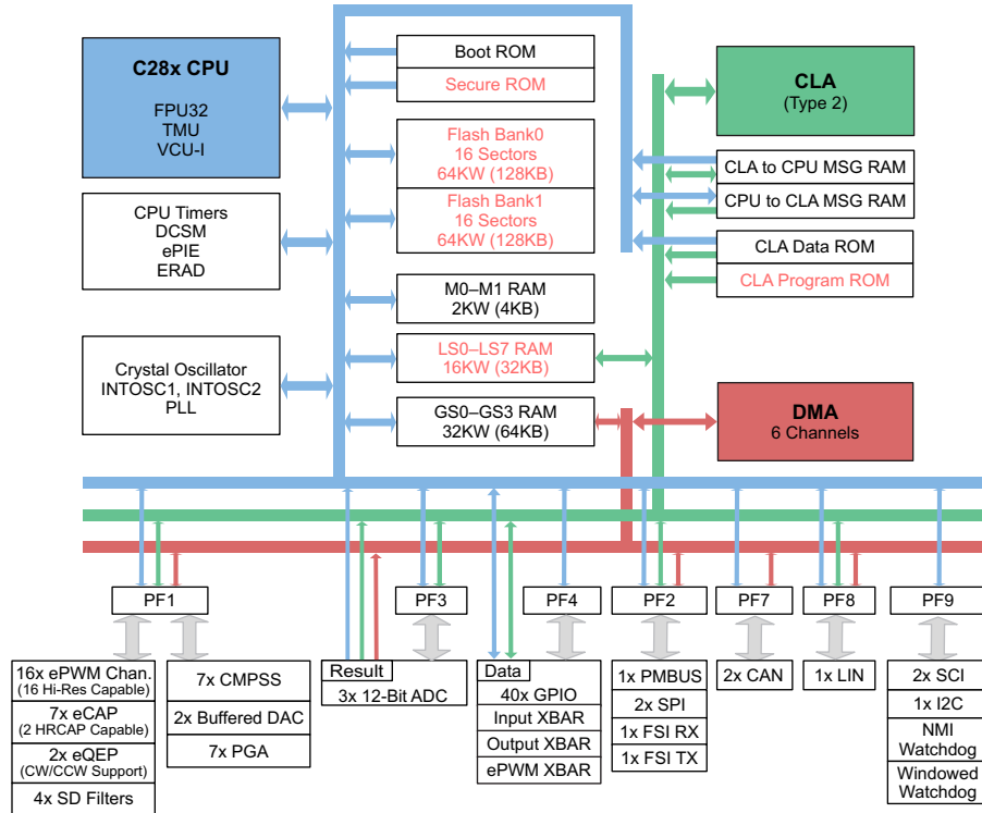
图 1-1. 功能方框图
