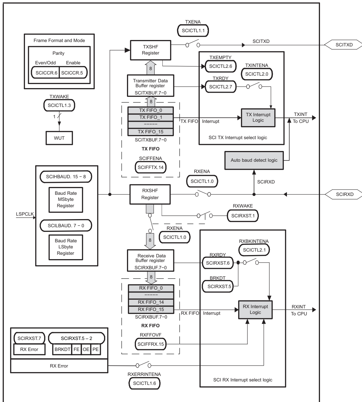
图 5-73. SCI Block Diagram
