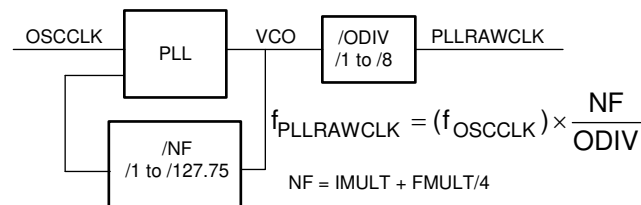
图 5-11. System PLL
