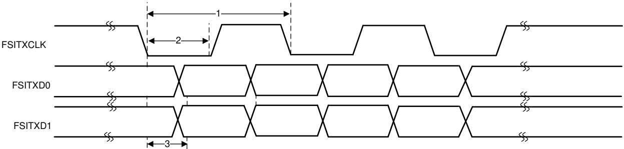
图 5-86. FSITX Timings
