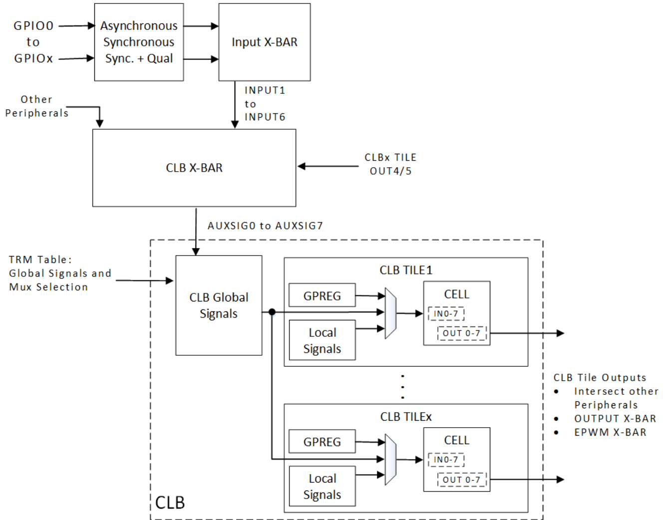
图 6-5. CLB Overview
