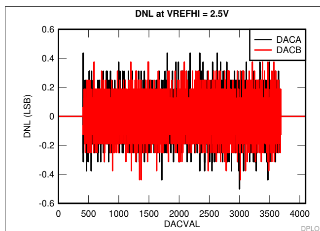
图 5-42. DNL
