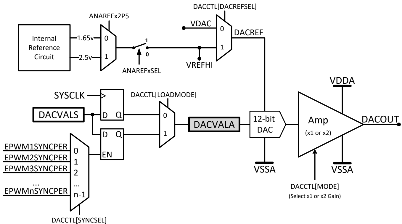
图 5-38. DAC Module Block Diagram
