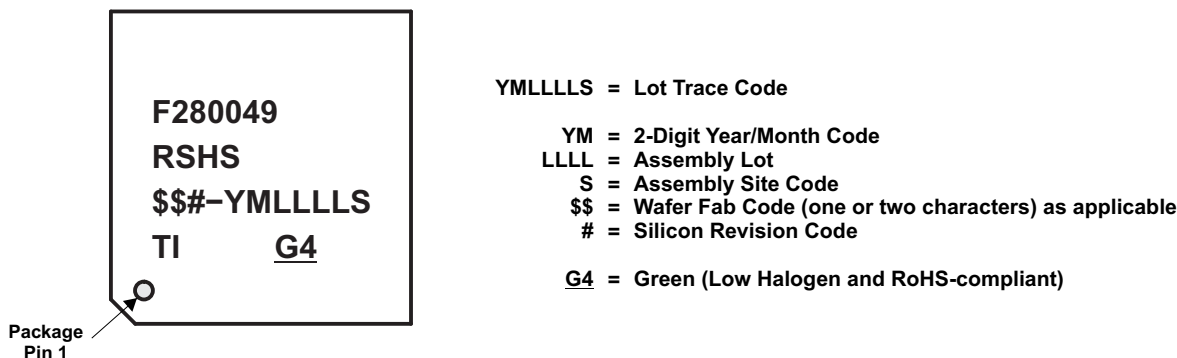
图 8-3. RSH 封装的器件标记示例
