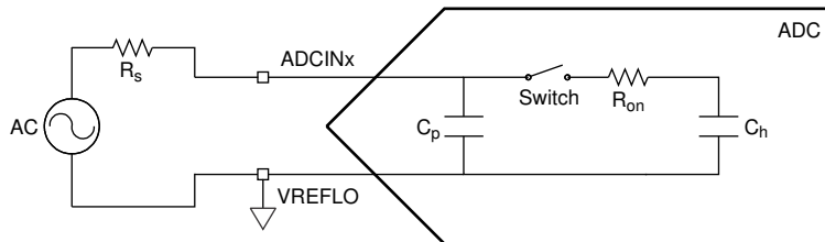
图 5-34. Input Model
