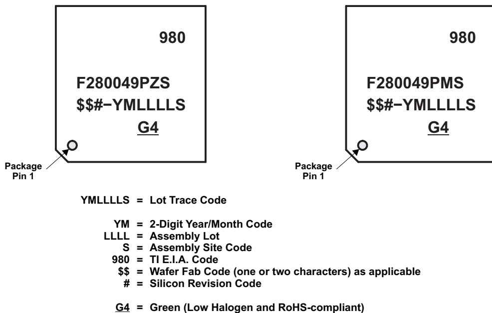
图 8-2. PM 和 PZ 封装的器件标记示例
