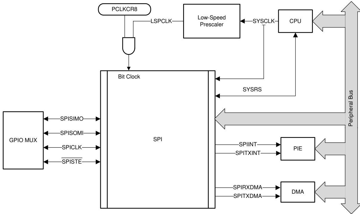
图 5-74. SPI CPU Interface
