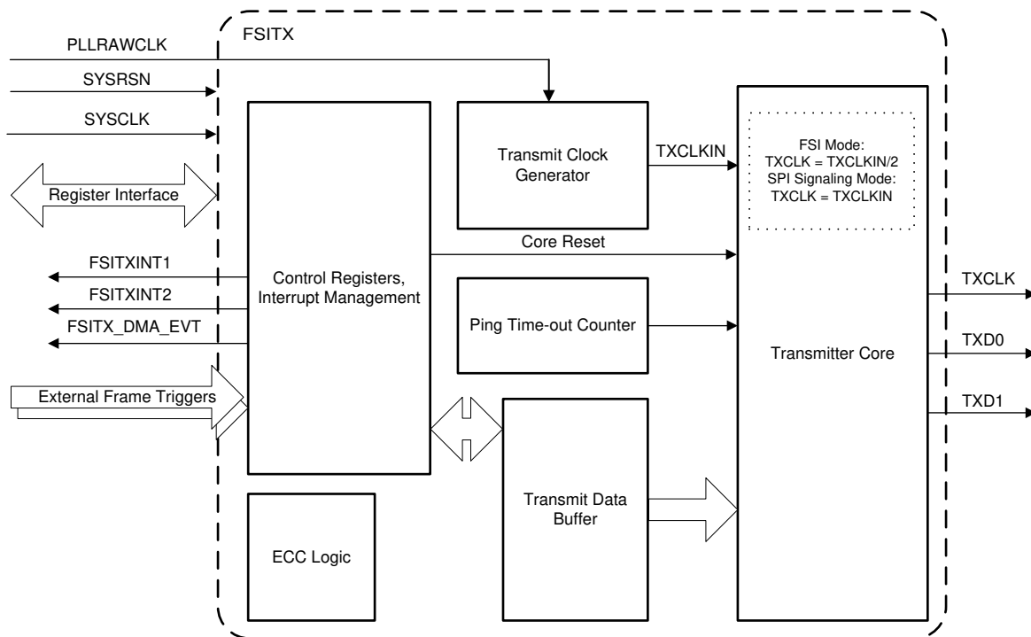
图 5-85. FSITX Block Diagram
