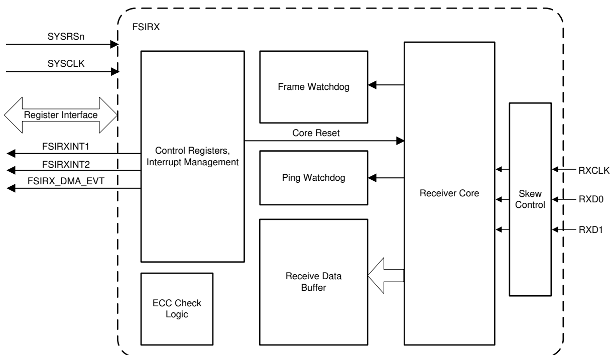
图 5-88. FSIRX Block Diagram
