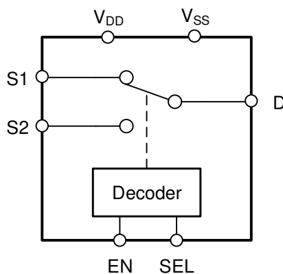
方框图
