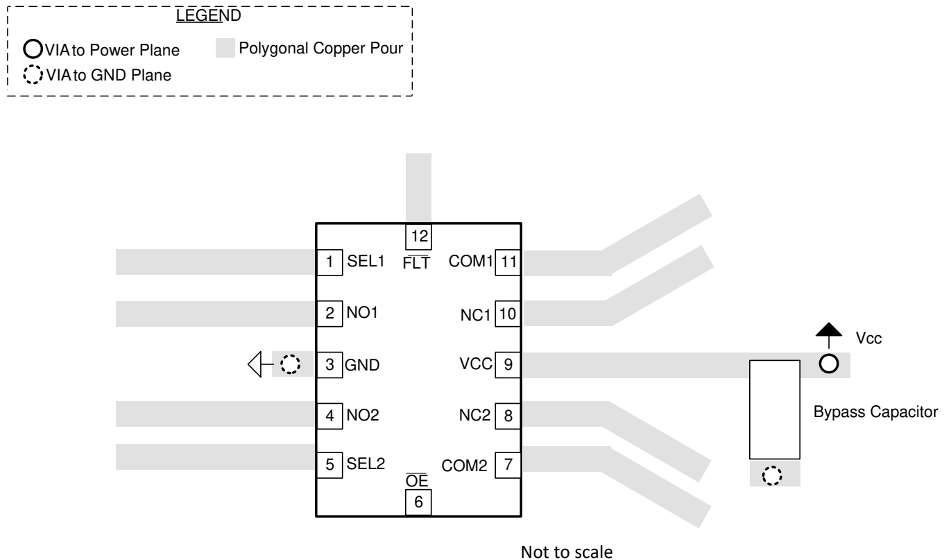
图 20. Layout Example
