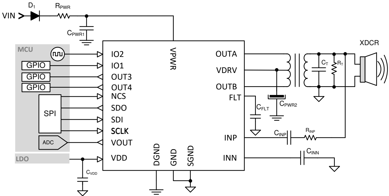
图 24. TUSS4440 Application Diagram
