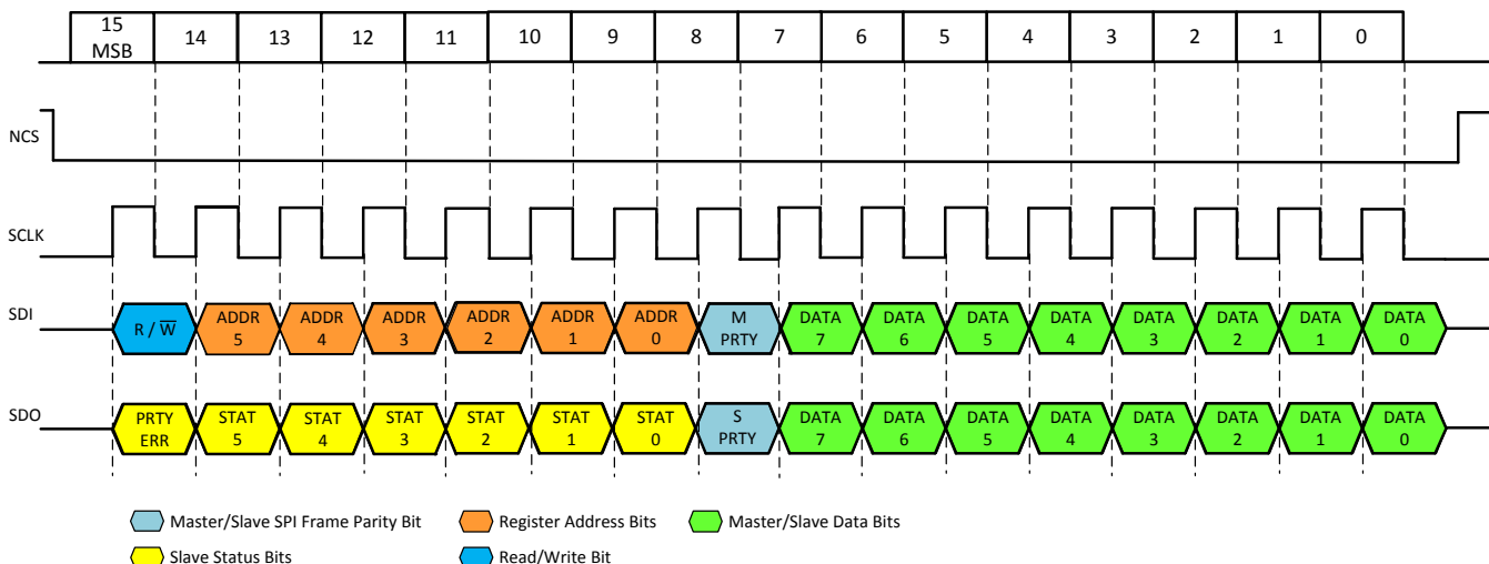
图 22. 16-Bit SPI Frame
