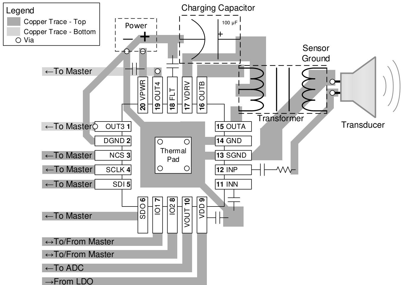
图 32. TUSS4440 Layout Example
