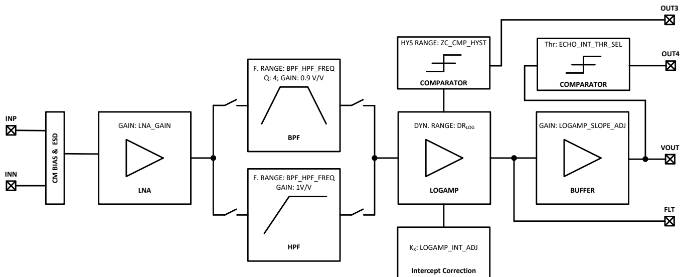
图 20. TUSS4440 Analog Front-End Block Diagram
