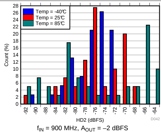
图 44. HD2 Histogram at AVDD19 = 1.9 V
