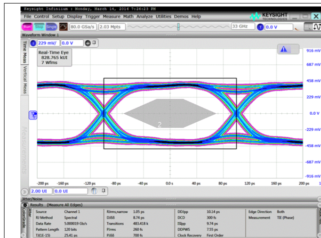
图 123. Data Eye at 5 Gbps
