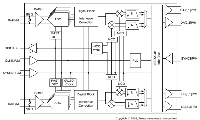
简化框图
