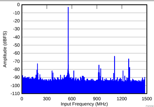
图 11. FFT for 2600-MHz Input Signal
