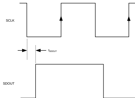
图 136. SDOUT Timing
