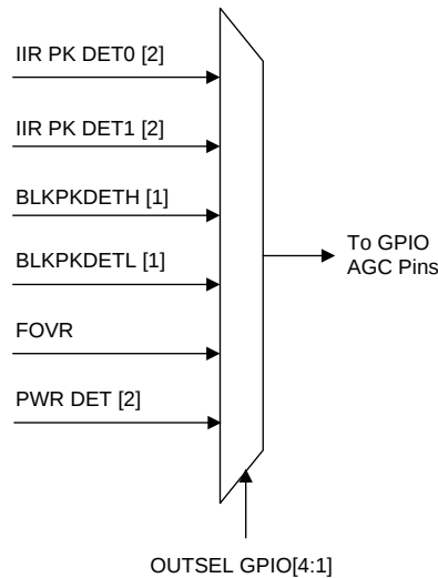
图 130. GPIO Output MUX Implementation
