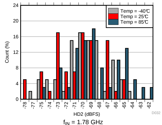
图 56. HD2 Histogram at AVDD19 = 1.9 V
