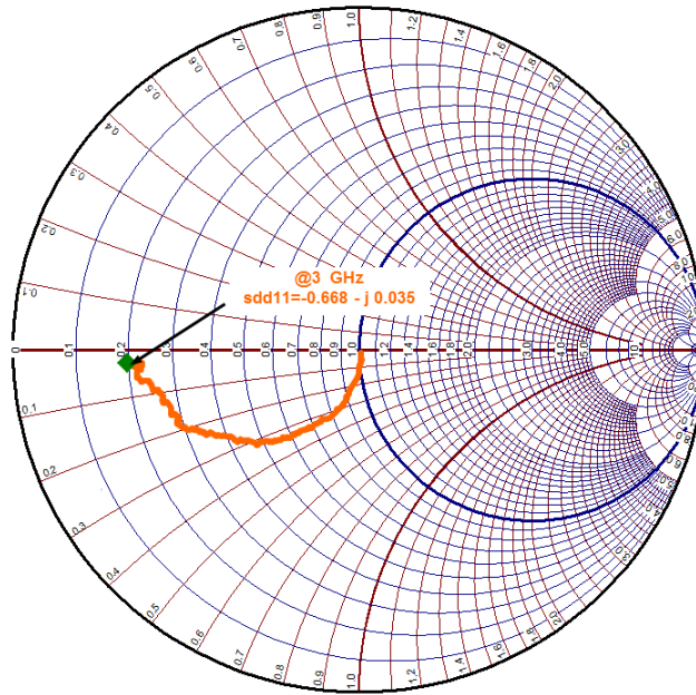
图 87. SDD11 of the Clock Input
