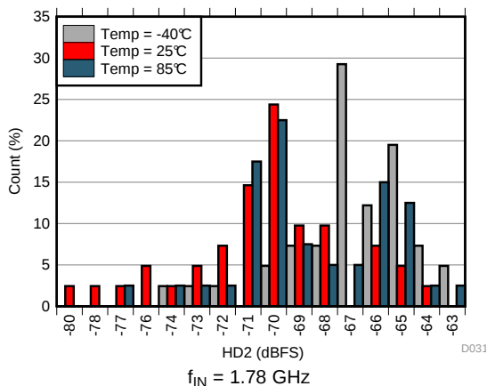
图 55. HD2 Histogram at AVDD19 = 1.8 V
