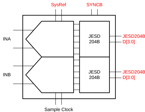
图 132. JESD Signal Overview
