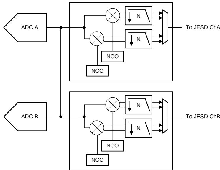
图 120. Digital Multiplexer Option
