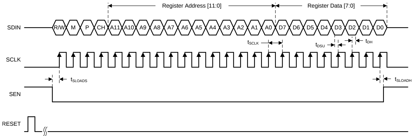
图 135. SPI Timing Diagram
