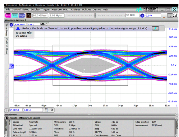
图 124. Data Eye at 12 Gbps
