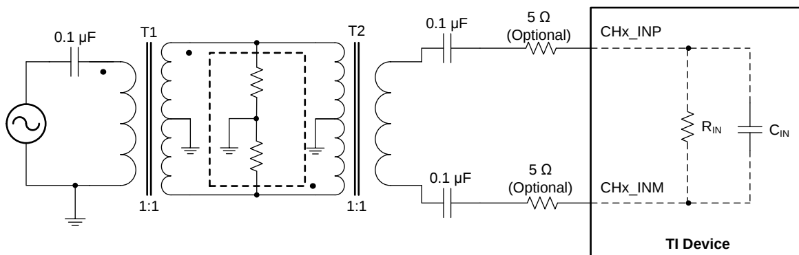
图 262. Input Drive Circuit
