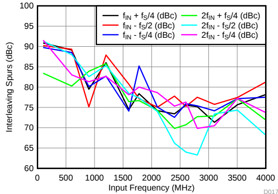
图 39. IL Spur vs Input Frequency
