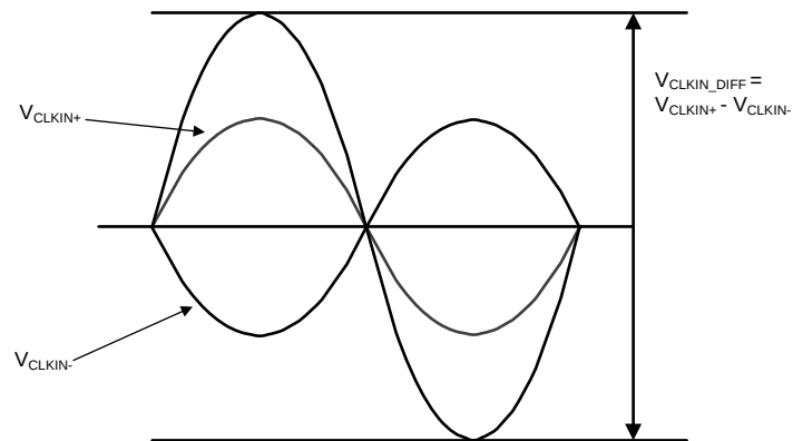
图 79. Input Clock Diagram
