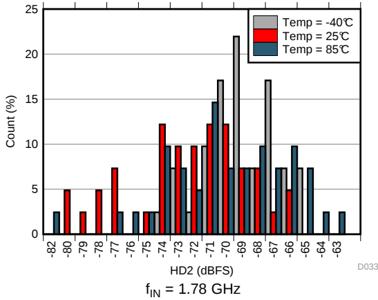
图 57. HD2 Histogram at AVDD19 = 2.0 V
