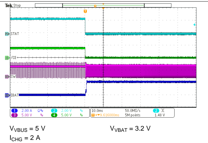
图 37. Charge Enable
