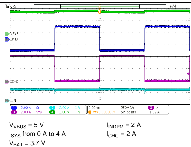
图 47. System Load Transient
