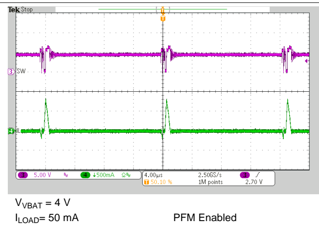
图 39. OTG Switching
