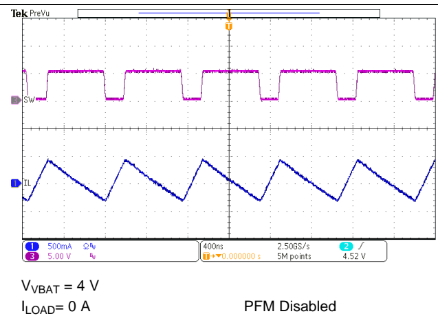
图 39. OTG Switching
