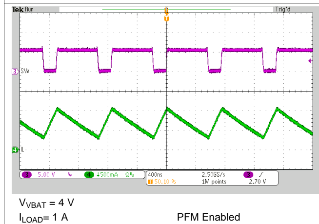
图 40. OTG Switching
