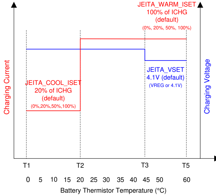
图 14. JEITA Profile
