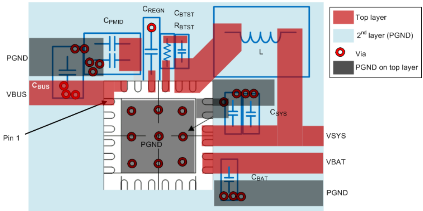
图 50. Layout Example
