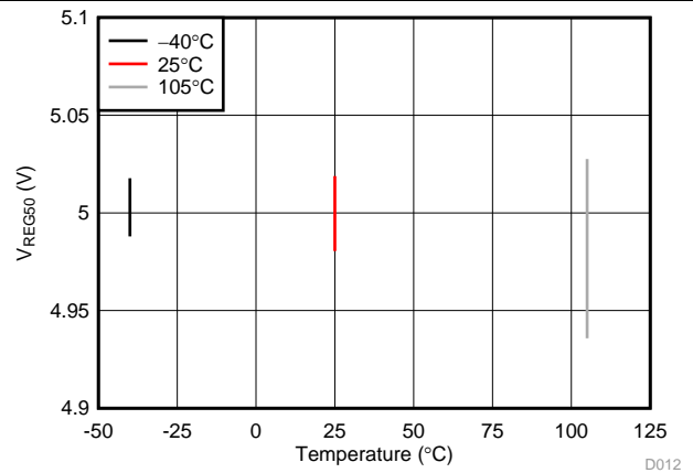
图 9. REG50 Output Voltage
