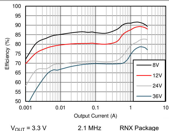
图 8-10. Efficiency
