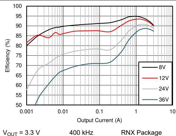
图 8-6. Efficiency
