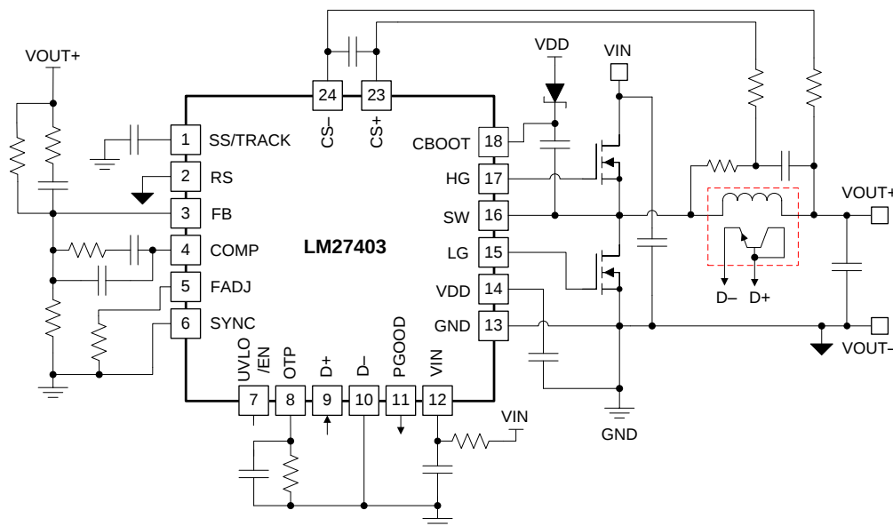
典型应用图
