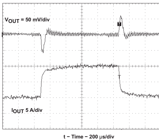
图 20. Transient Response
