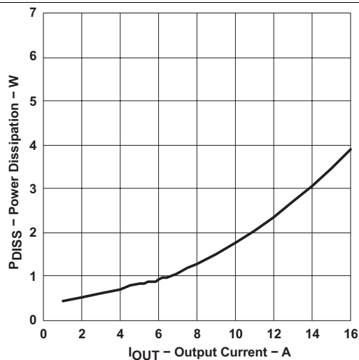
图 17. Power Dissipation vs. Load
