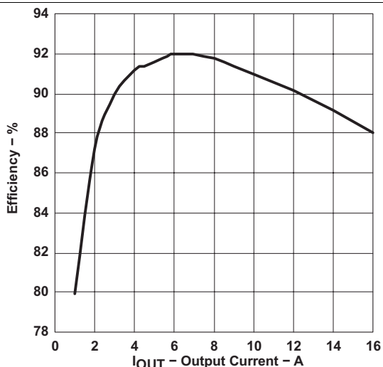
图 16. Efficiency vs. Load
