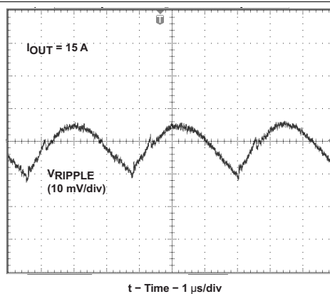
图 19. Output Voltage Ripple
