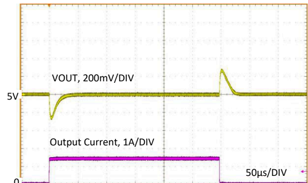
图 9-27. Load Transient
