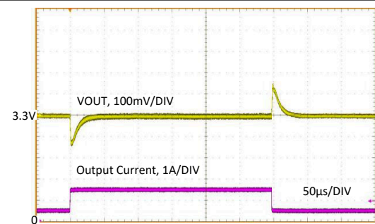
图 9-29. Load Transient
