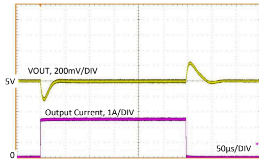
图 9-26. Load Transient
