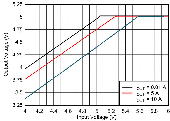
图 9-24. Dropout
