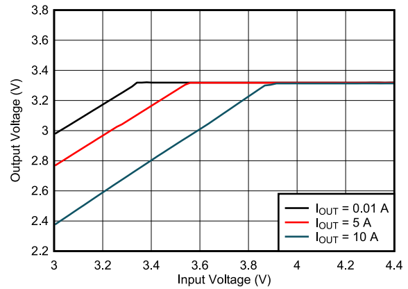
图 9-25. Dropout
