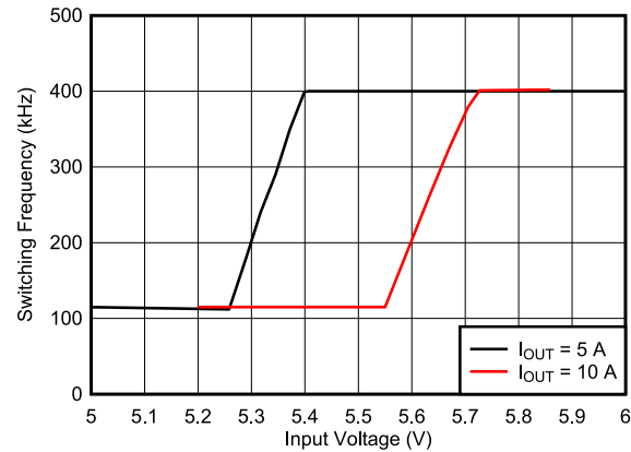
图 9-24. Dropout
