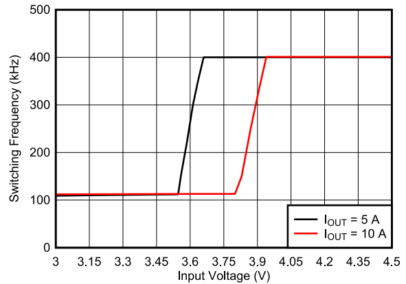
图 9-25. Dropout
