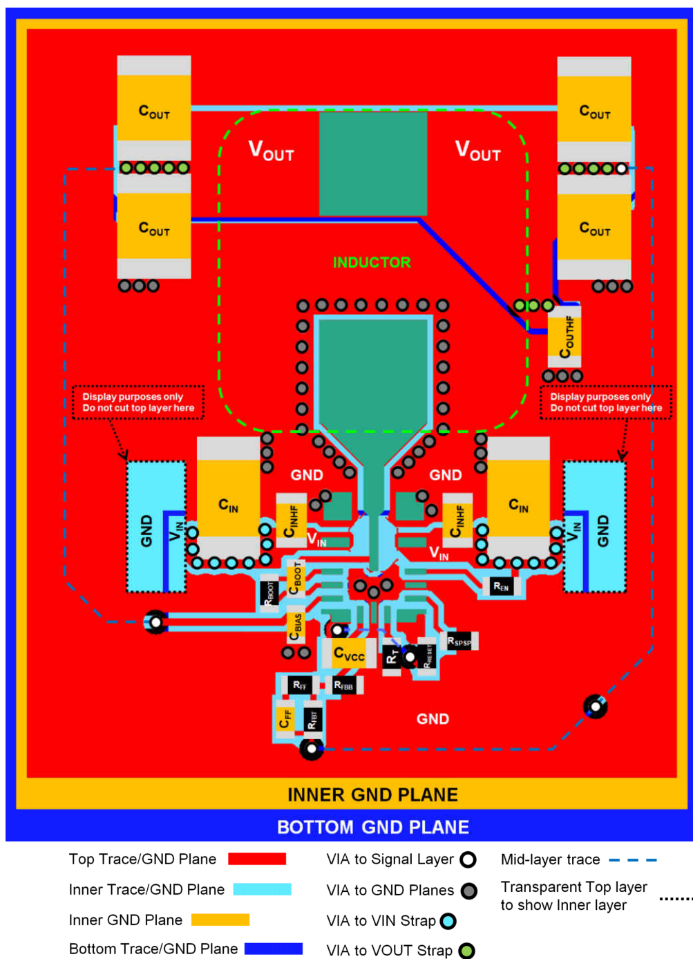
图 11-2. Layout Example
