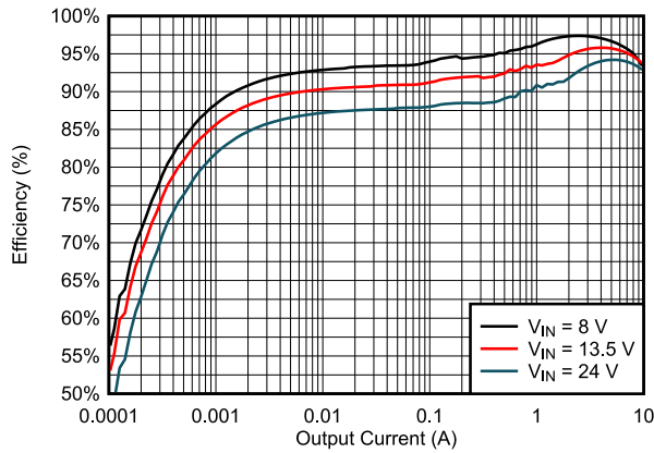
图 9-6. Efficiency
