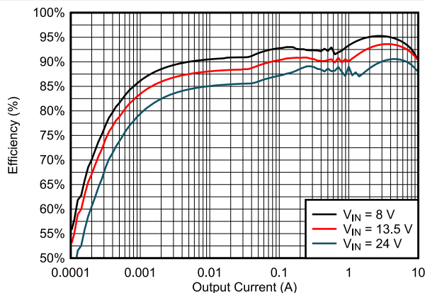
图 9-8. Efficiency
