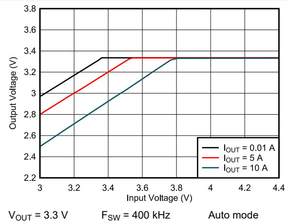
图 9-23. Dropout
