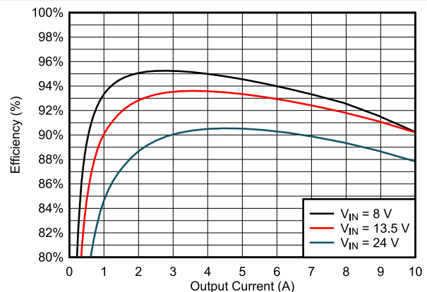
图 9-9. Efficiency
