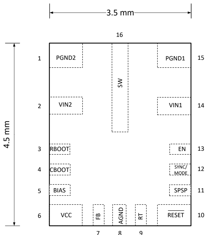
图 6-1. RPH Package 16-Pin VQFN (Top View)
