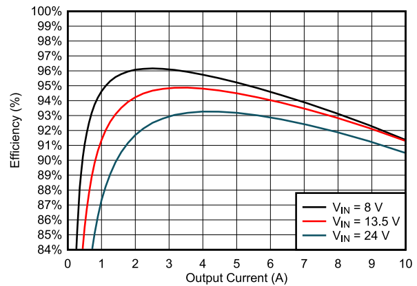
图 9-7. Efficiency
