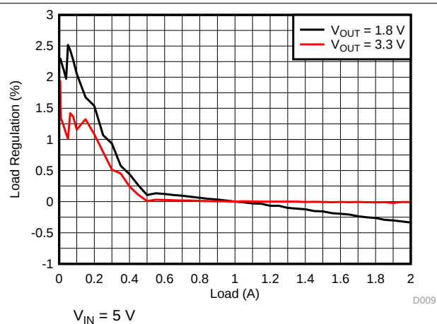
图 10. Load Regulation
