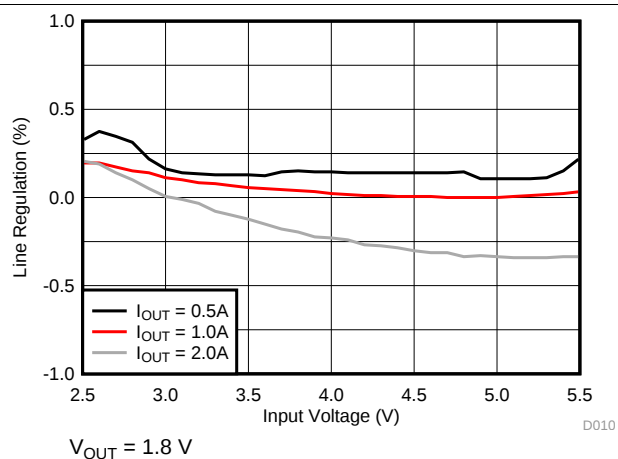
图 11. Line Regulation
