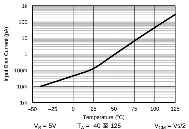
Figure 6. 输入偏置电流与温度间的关系
