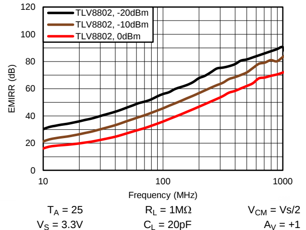
Figure 36. EMIRR 性能
