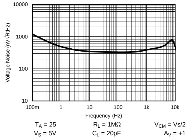
Figure 34. 输入电压噪声与频率间的关系
