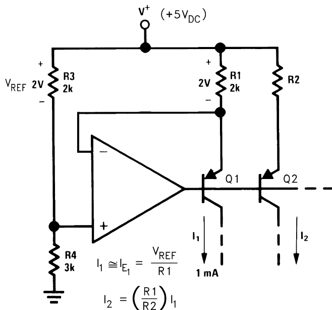
Figure 67. 固定拉电流
