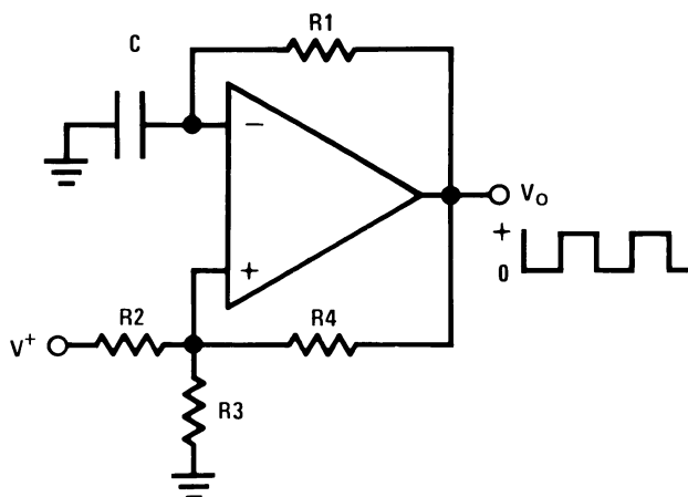
Figure 66. 方波发生器
