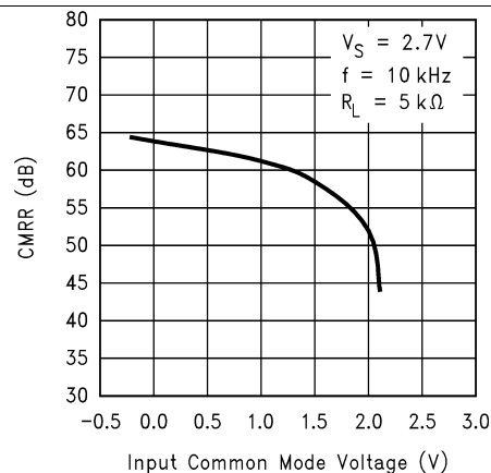
Figure 14. CMRR 与输入共模电压间的关系
