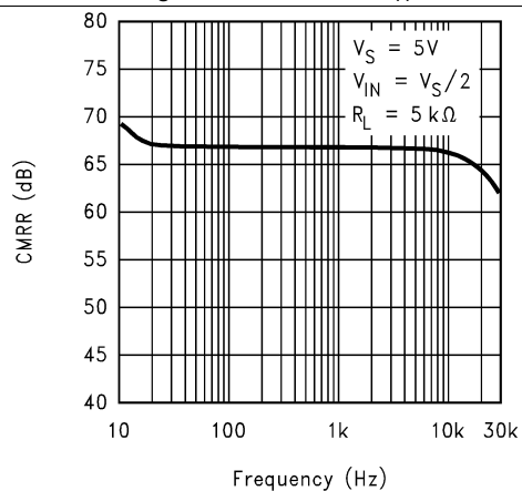
Figure 13. CMRR 与频率间的关系
