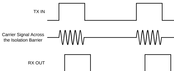
图 43. OOK-Based Modulation Scheme
