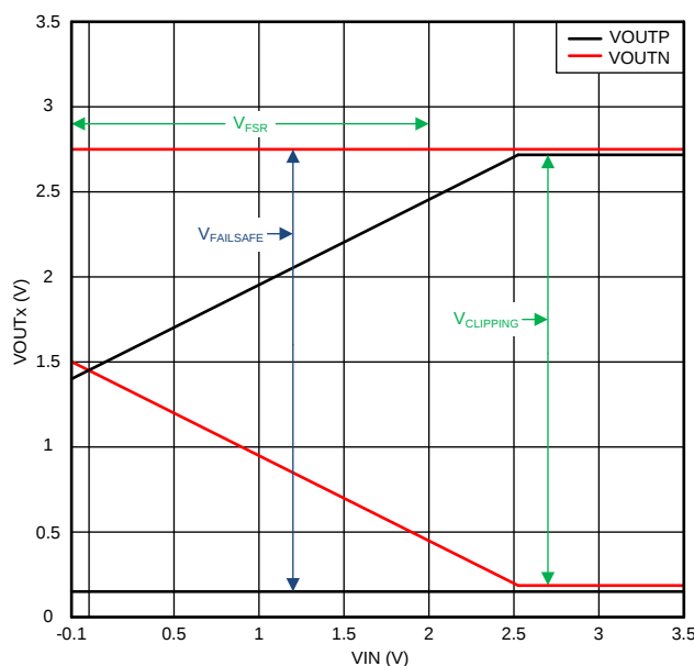
图 44. AMC1211A-Q1 Output Behavior
