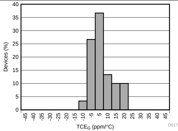
图 17. Gain Error Drift Histogram
