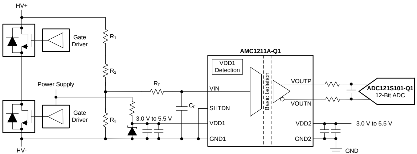
简化原理图
