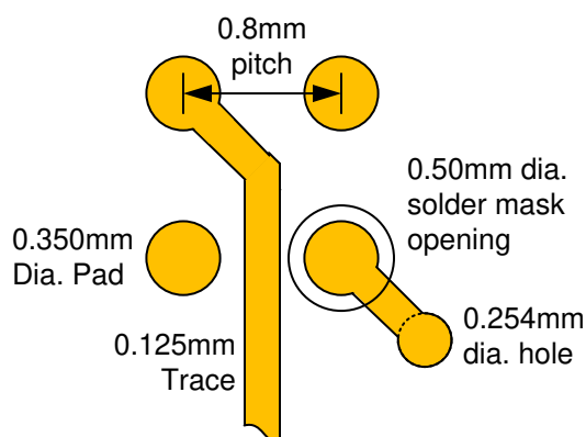
图 12-1. BGA Layout Example
