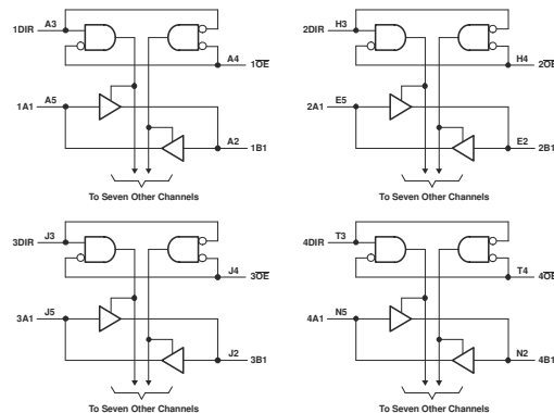
图 3-1. 逻辑图
