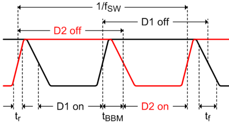
图 35. Timing Diagram
