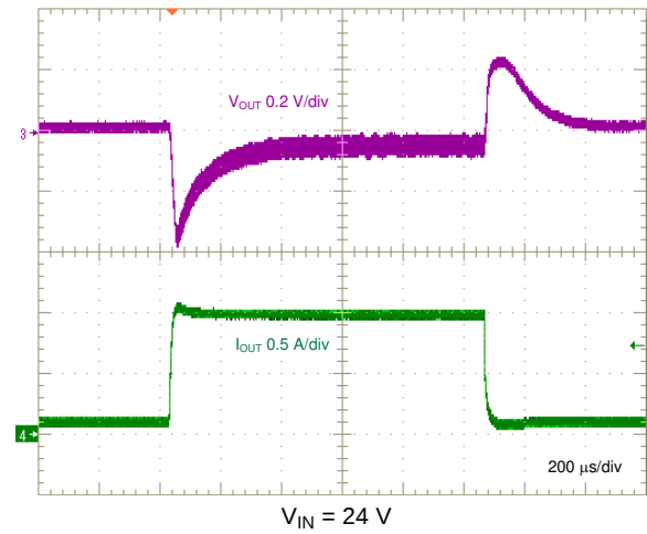
图 29. Load Transient, 0.1 A to 1 A, 0.1 A/ \mu\text{s}
