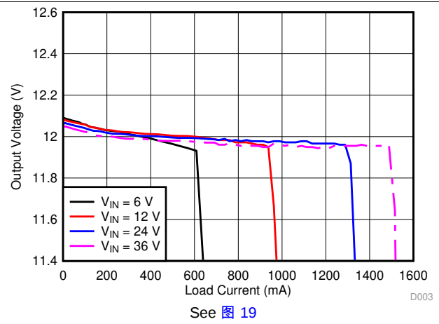
图 2. Output Voltage versus Load
