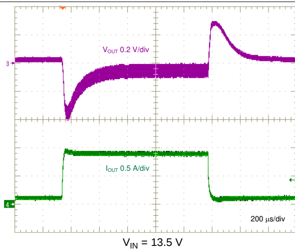
图 30. Load Transient, 0.1 A to 1 A, 0.1 A/ \mu\text{s}
