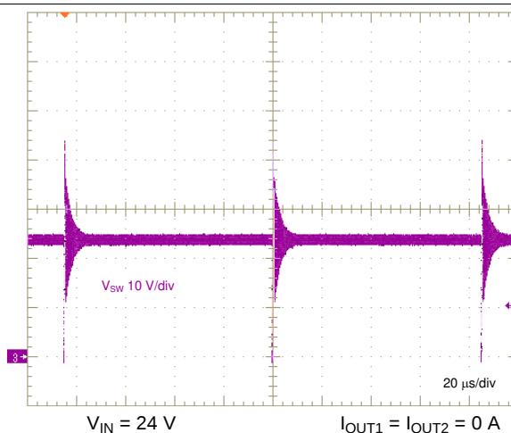
图 40. Switch Voltage, No Load
