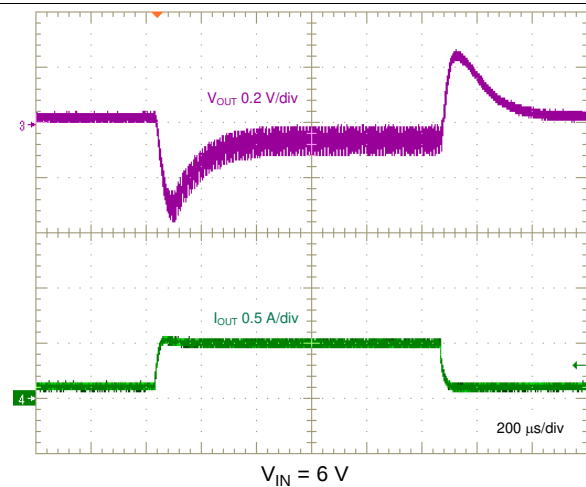
图 31. Load Transient, 0.1 A to 0.5 A, 0.1 A/ \mu\text{s}
