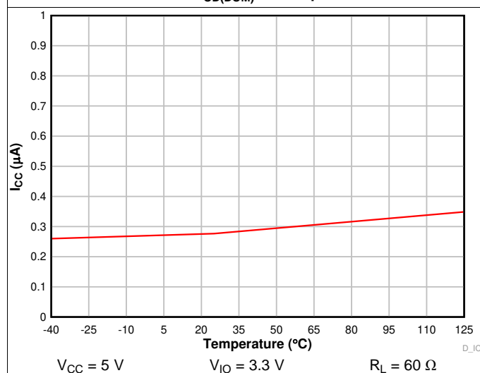
图 3. I_{CC} Standby vs Temperature
