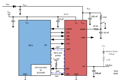
简化电路原理图, SPI 模式
