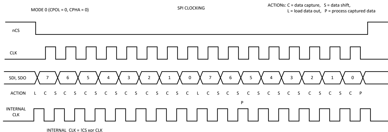
图 35. SPI Clocking
