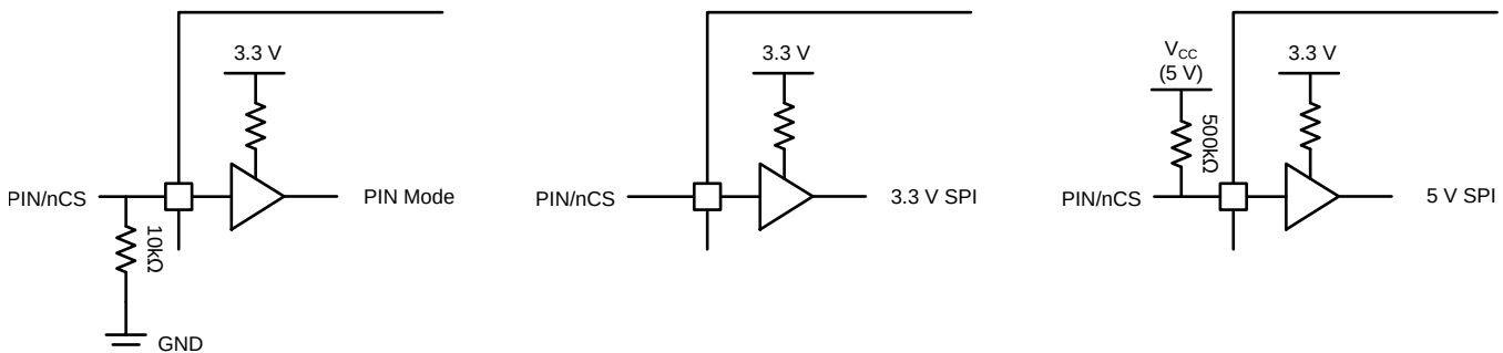
图 29. PIN/nCS Configuration
