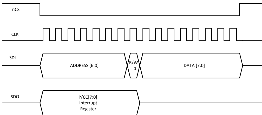
图 36. SPI Write
