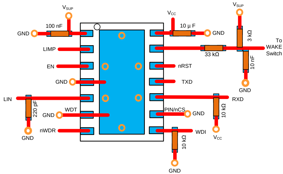
图 51. Layout Example
