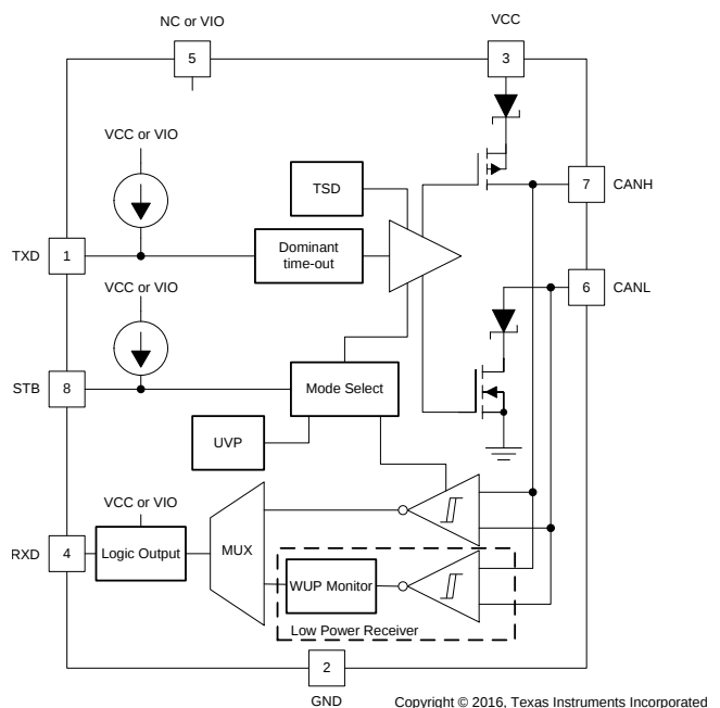
功能框图
