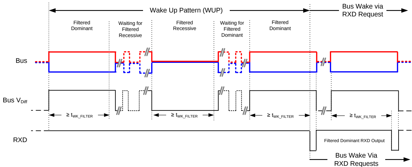
图 15. Wake Up Pattern (WUP)
