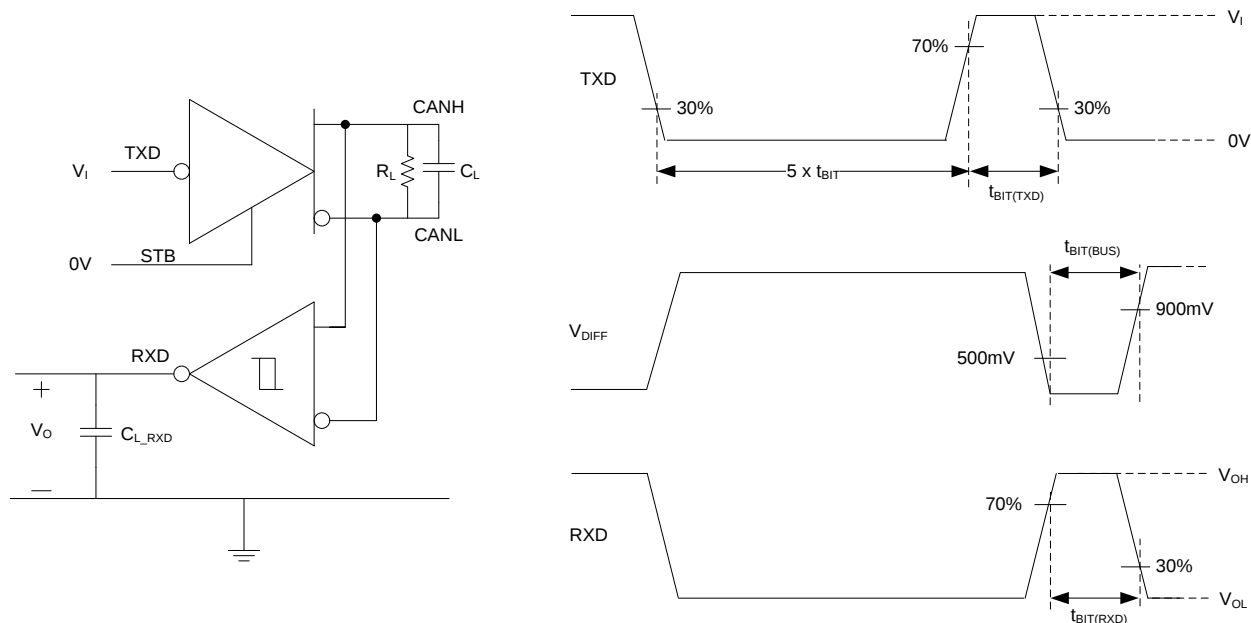
图 9. CAN FD Timing Parameter Measurement
