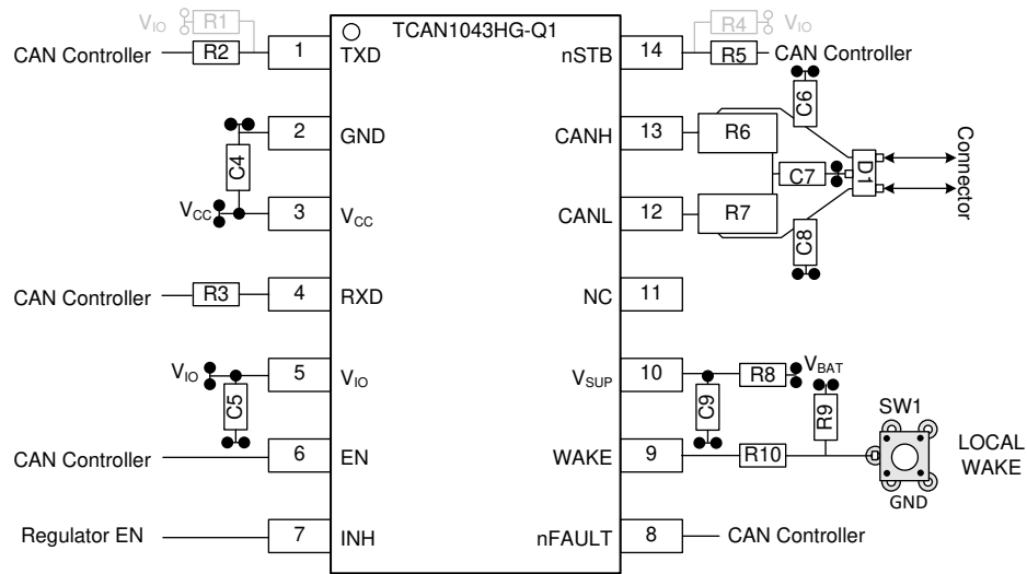
图 31. TCAN1043xx-Q1 Layout Example
