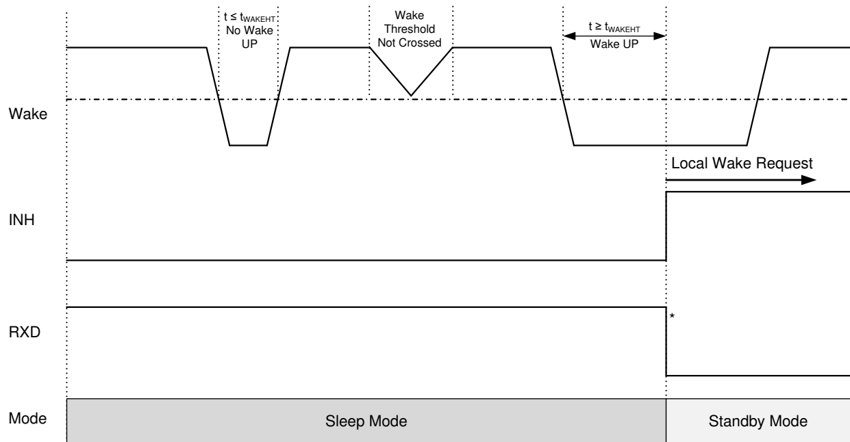
图 25. Local Wake Up – Falling Edge
