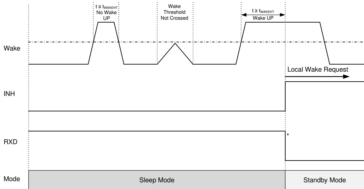
图 24. Local Wake Up – Rising Edge
