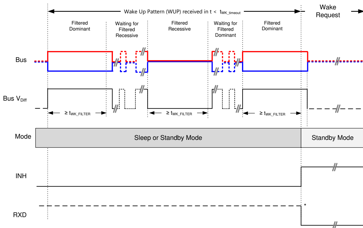
图 22. Wake Up Pattern (WUP)
