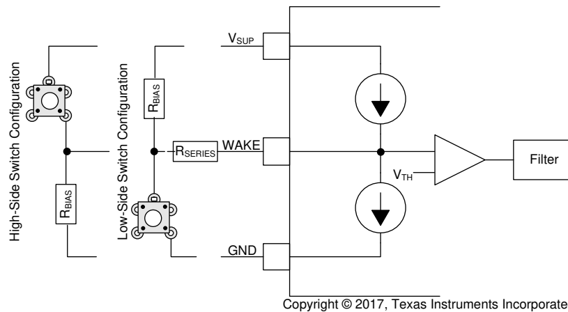
图 23. TCAN1043xx-Q1 WAKE Circuit Example
