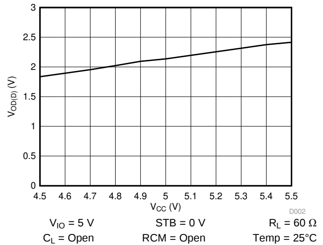
图 2. V_{OD(D)} over V_{CC}
