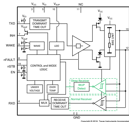
功能方框图
