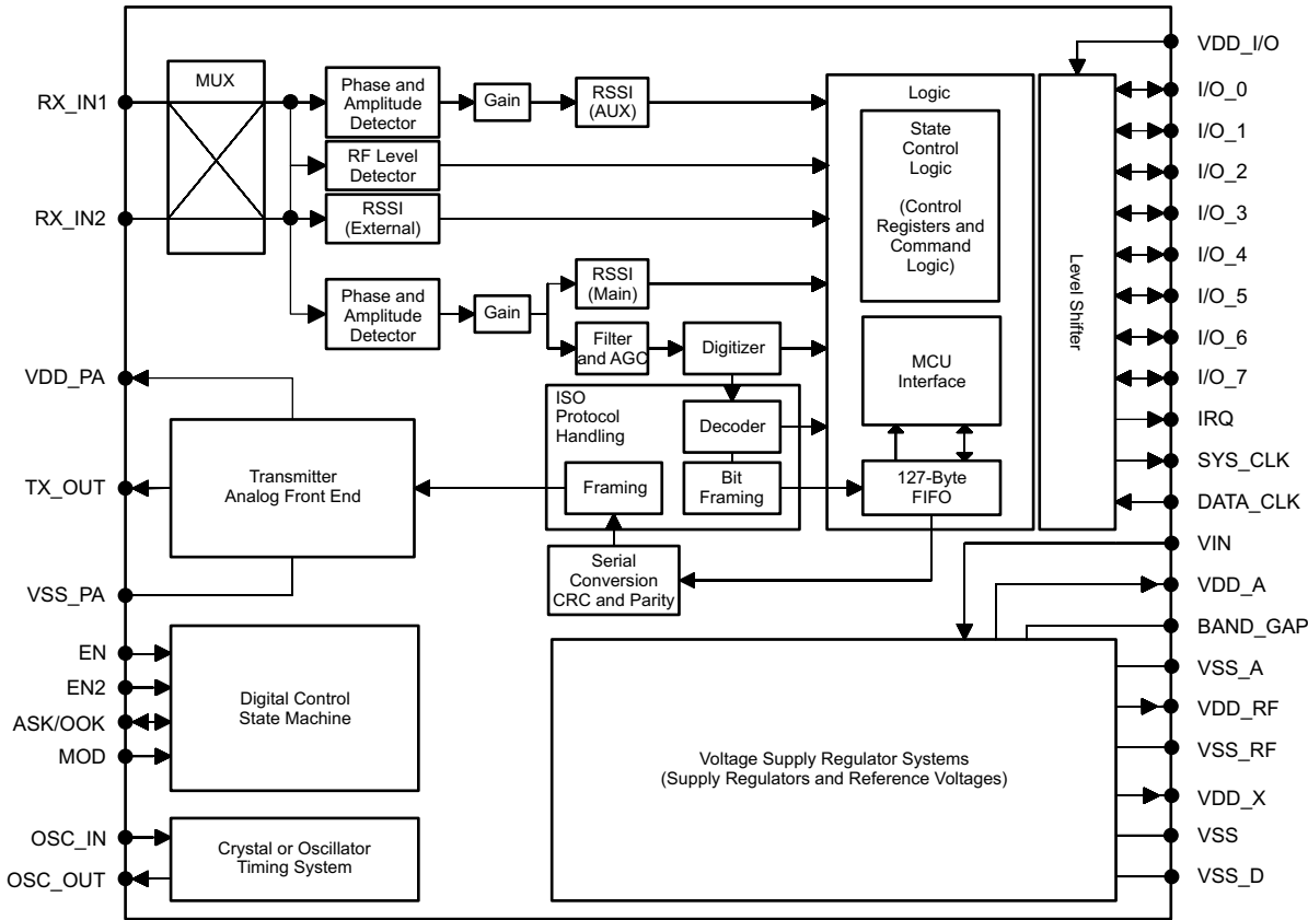
图 1-1. 方框图
