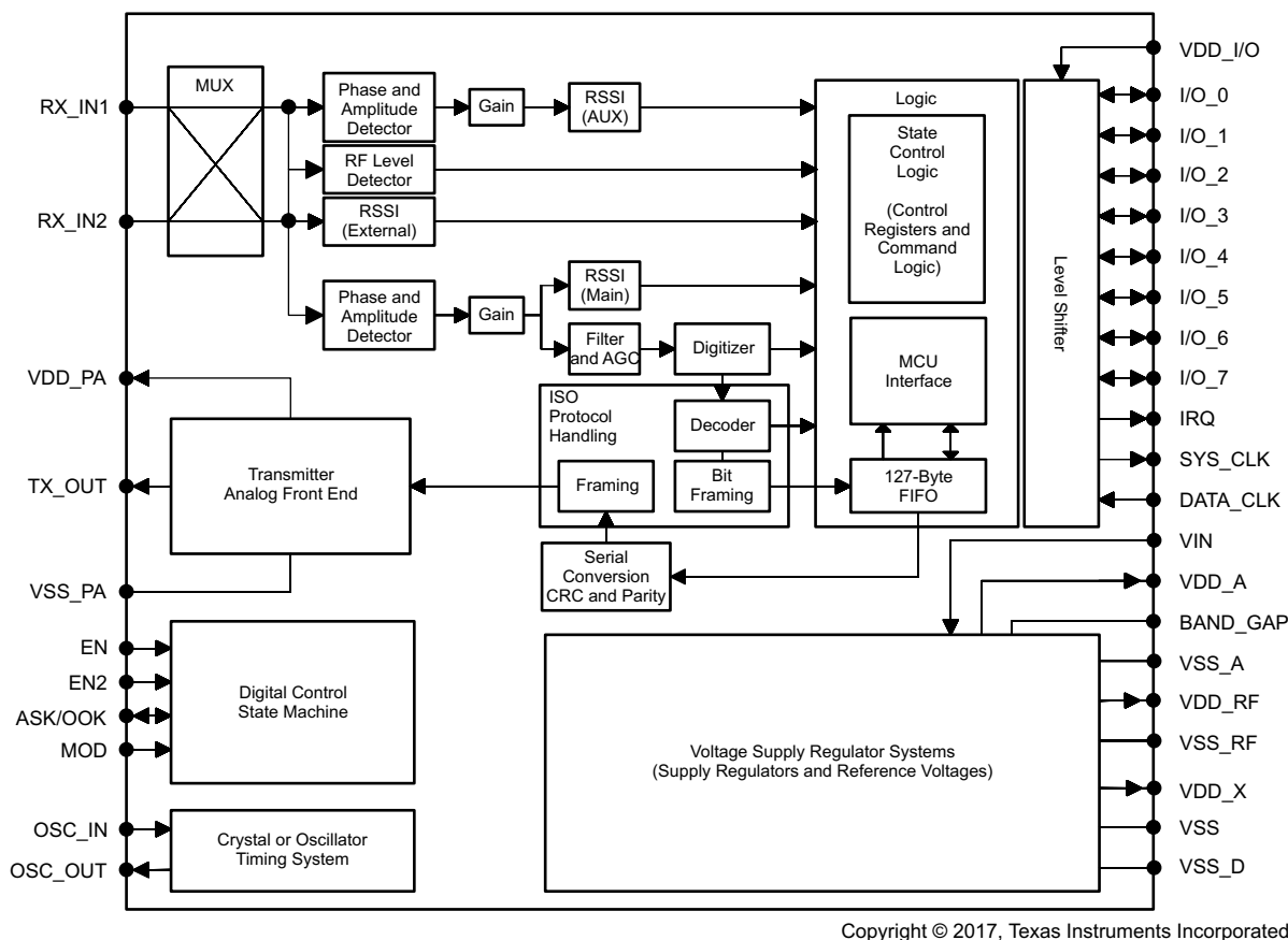
图 6-2. System Block Diagram
