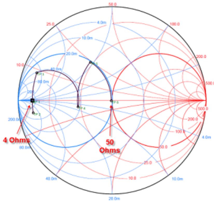
图 7-3. Smith Chart Simulation
