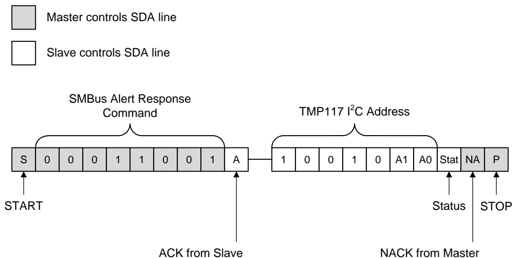
图 24. SMBus ALERT Timing Diagram
