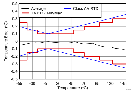
DRV 温度精度
