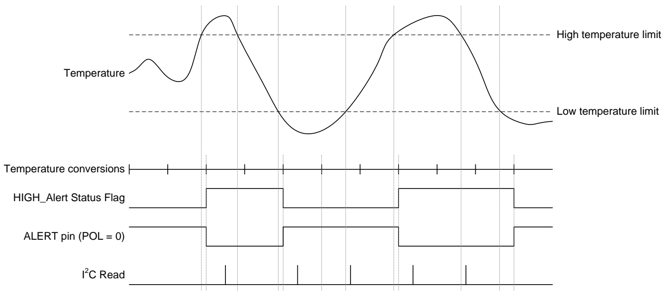
图 19. Therm Mode Timing Diagram
