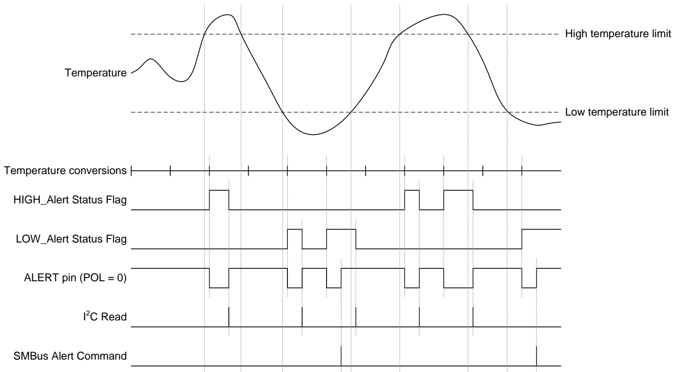
图 18. Alert Mode Timing Diagram
