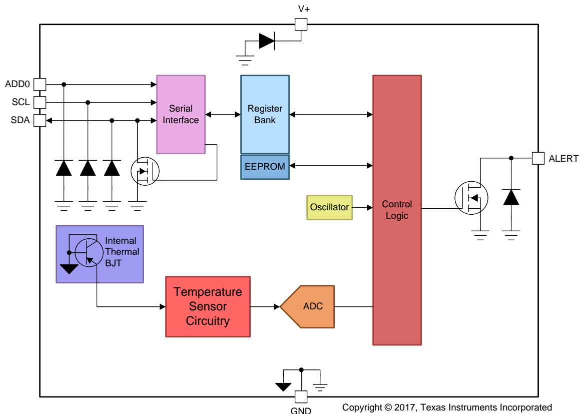
图 14. Internal Block Diagram
