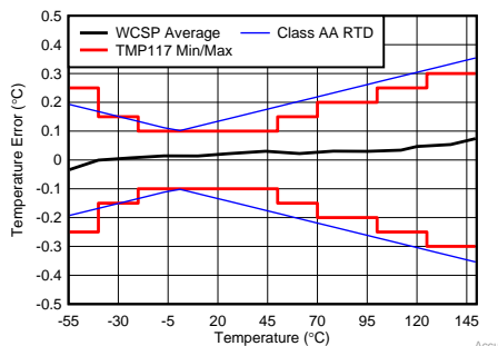
YBG 温度精度
